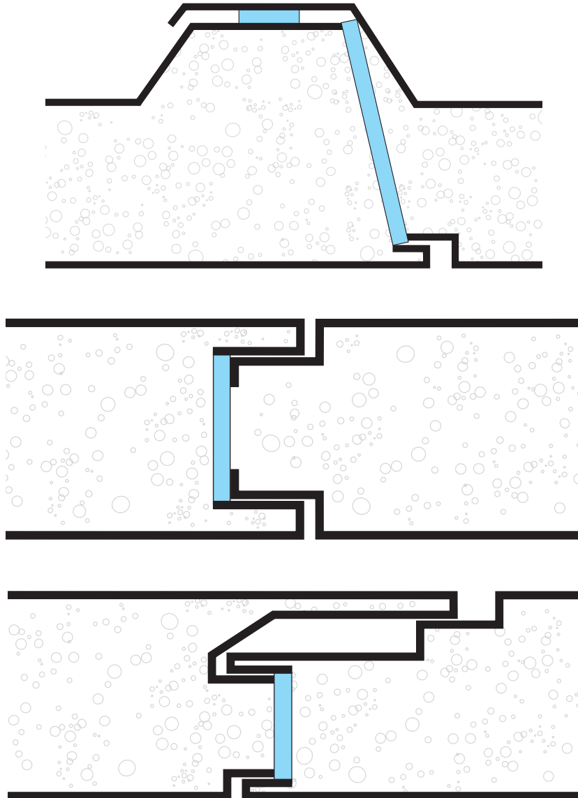
Figure 26 : joints de bardage en panneaux sandwichs
