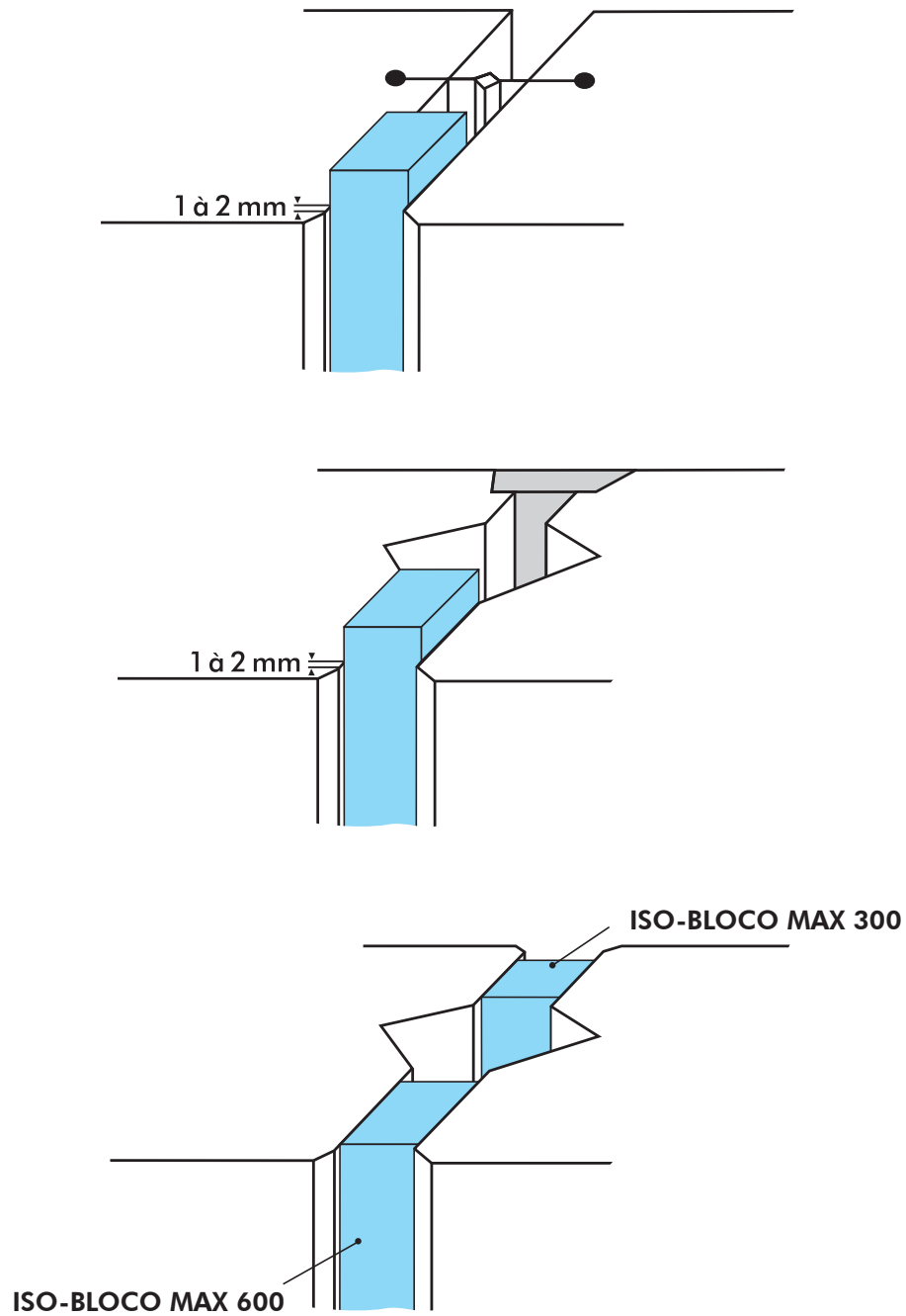
Figure 20 : en partie verticale d'éléments préfabriqués lourds
